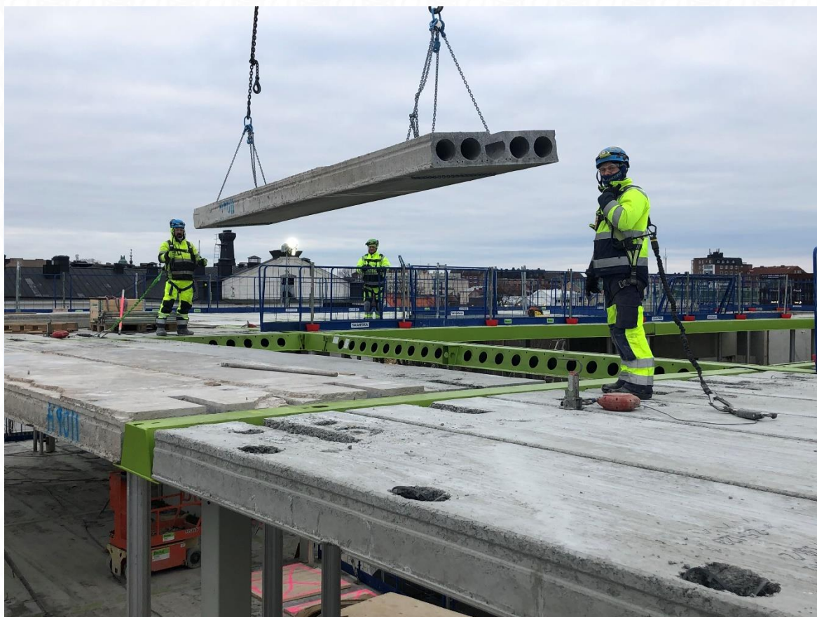
Foto: Montage av håldäcksbjälklag i projekt Skeppsbrokajen , Karlskrona
